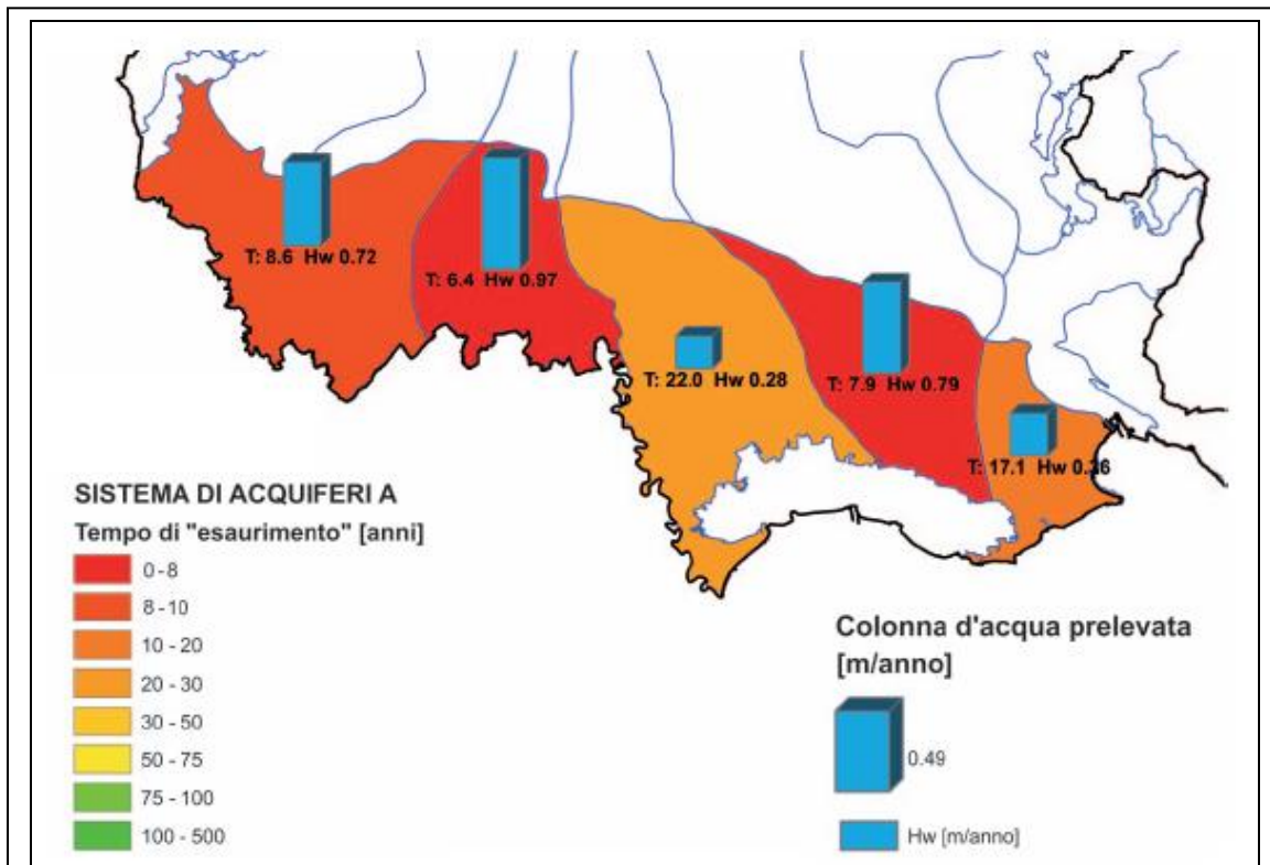
Figura 127 - Tempo di esaurimento sistema di acquiferi A
