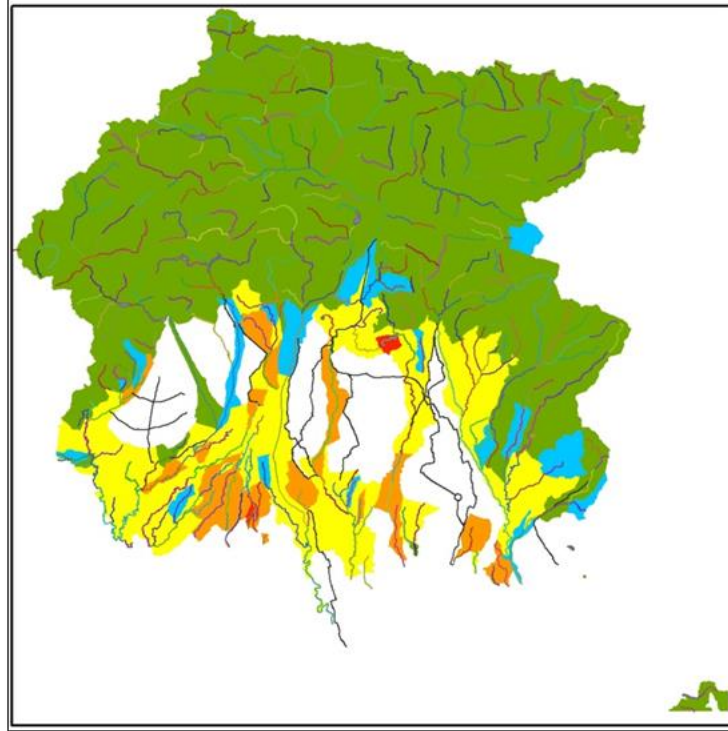
Figura 41 - Carta rappresentante le classi dell'indicatore uso agricolo del suolo.
