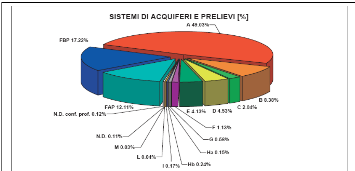
Figura 99 - Distribuzione dei prelievi per ciascun sistema di acquiferi di emunzione
