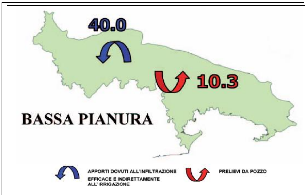
Figura 122 - La ricarica della falda freatica della Bassa Pianura. I prelievi in Bassa Pianura sono solamente quelli dalla falda freatica
