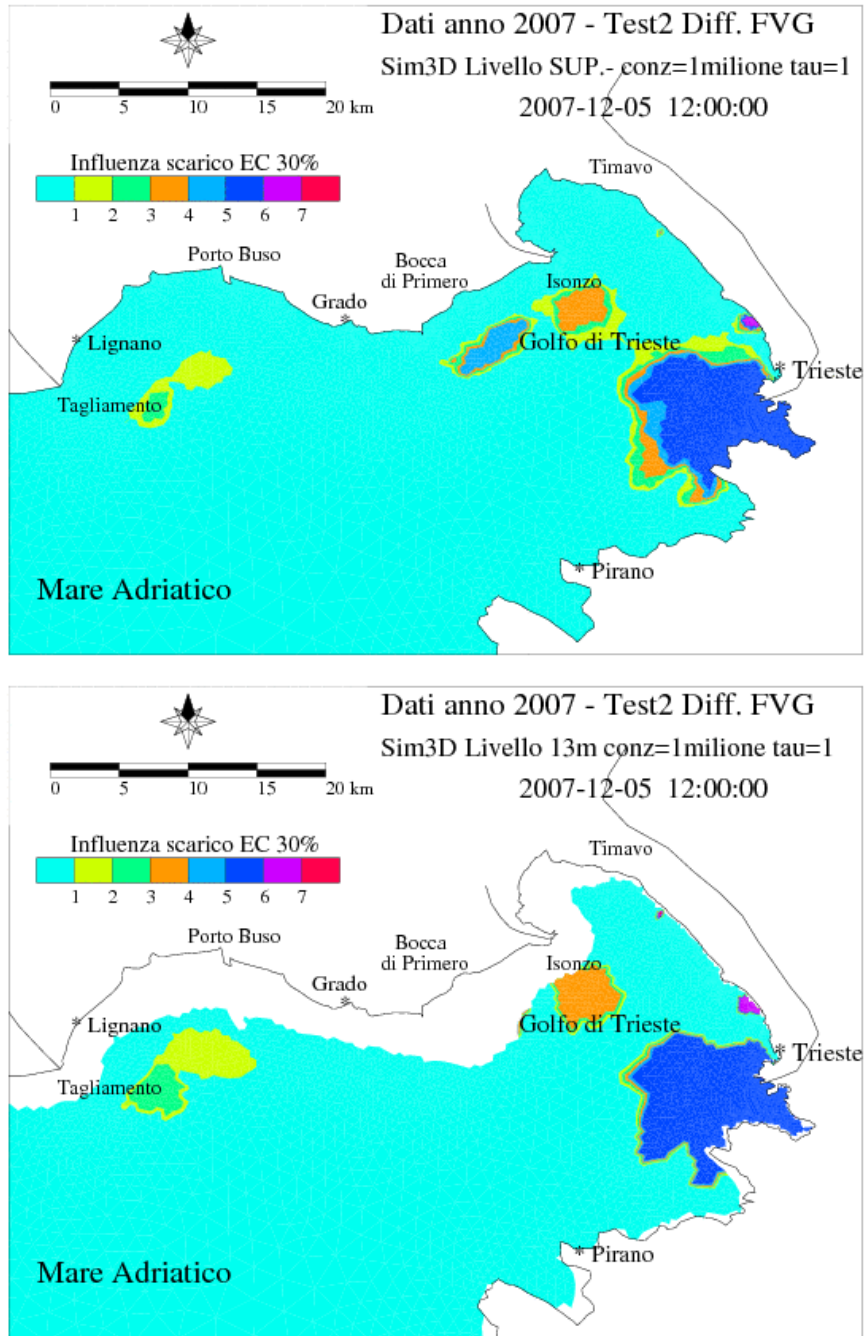
Figura 25 - Mappe dell'area di influenza delle 7 condotte sottomarine della regione per il giorno 5.12.2007 ore 12 - tempo di decadimento della carica batterica di 1 giorno e concentrazione in uscita di 1.000.000 UFC/100mL (tranne per i diffusori di Servola e Barcola). Sopra: mappa per il livello di superficie. Sotto: mappa del livello 13 metri.
