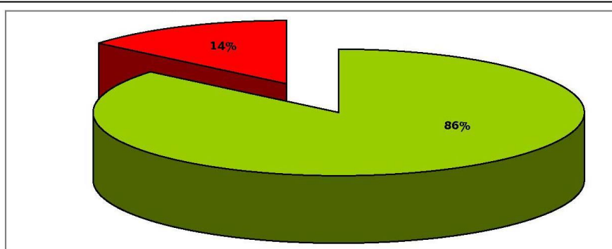
Figura 4- Classificazione di perennità. In rosso la percentuale di tratti temporanei, in verde la percentuale di tratti perenni
