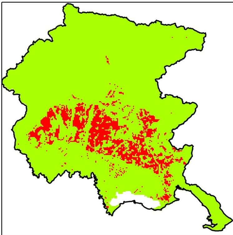
Figura 79 - acque sotterranee: risultati dell'analisi di significatività dell'indicatore surplus di azoto (in rosso le celle nelle quali la pressione risulta potenzialmente significativa)
