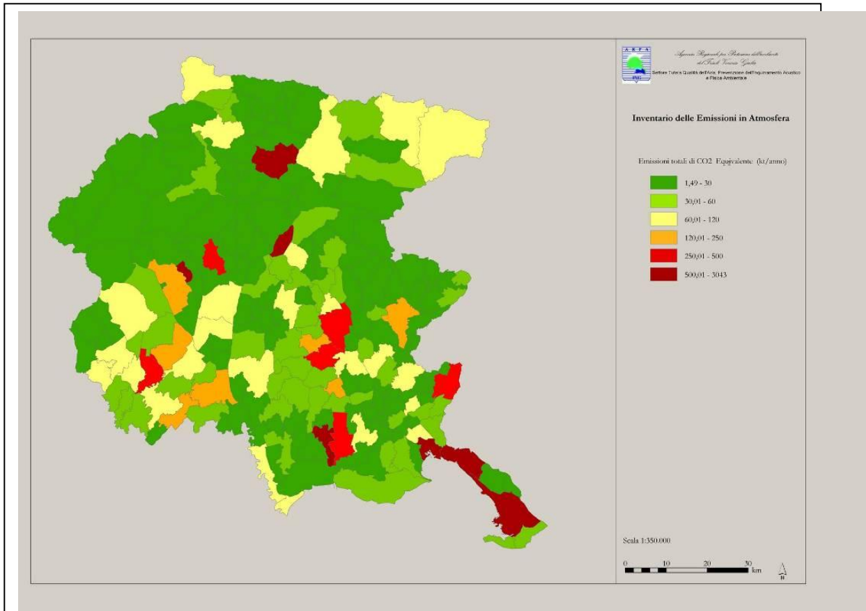
Figura 53 - Emissioni di sostanze CO 2 equivalenti (sostanze ad effetto serra) in atmosfera per i diversi Comuni del Friuli Venezia Giulia.
