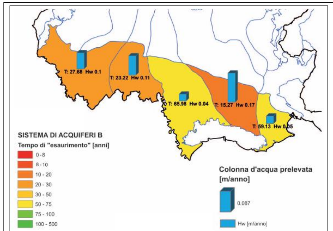
Figura 128 - Tempo di esaurimento sistema di acquiferi B
