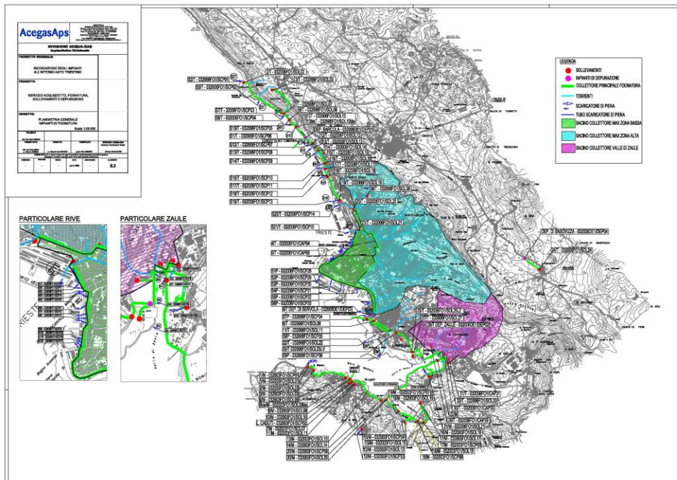
Figura 28 –Cartografia contenente la rete fognaria e l'ubicazione degli sfioratori di piena delle province di Udine (fonte Piano d'Ambito 2014 – figura in alto) e di Trieste (fonte Acegas – figura in basso). In provincia di Udine gli sfioratori di piena sono complessivamente 804 mentre in provincia di Trieste sono 44 tutti recapitanti in mare.
