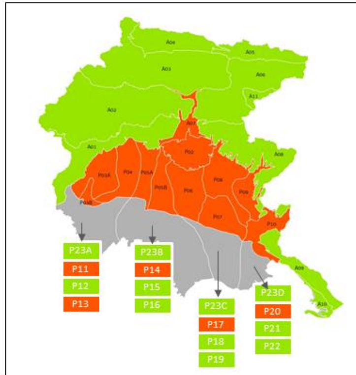
Figura 168 – Stato quantitativo dei corpi idrici sotterranei
